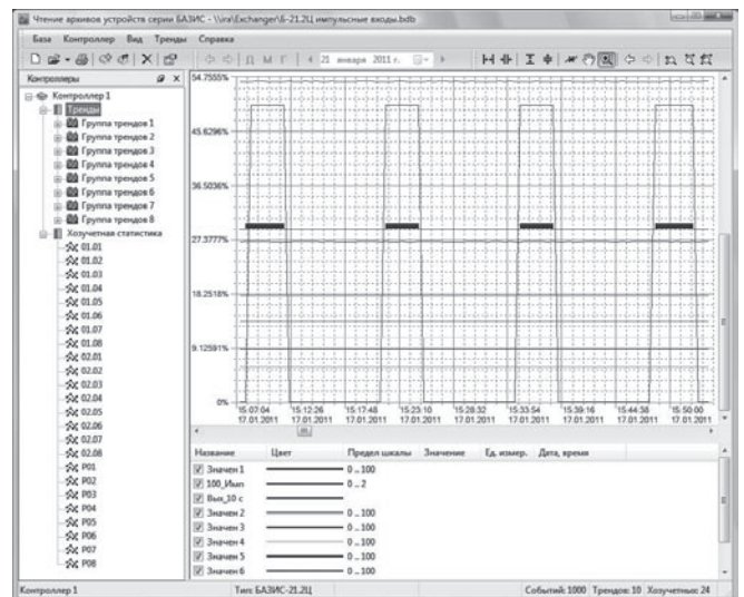
Рис. 2. Программа чтения архивов устройств серии БАЗИС
