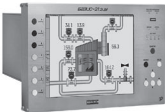
▲ Универсальный промышленный контроллер БАЗИС-21.2ЦУ
